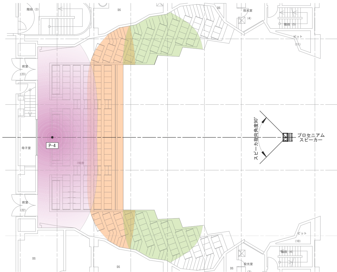
2階平面図
